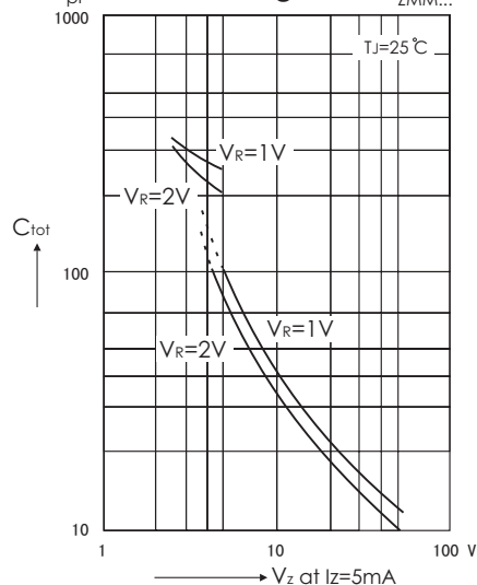
Capacitance versus Zener voltage
