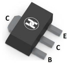
SOT-89
