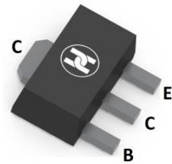
SOT-89
