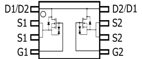
TSSOP-8
