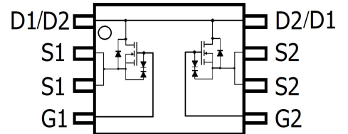
TSSOP-8
