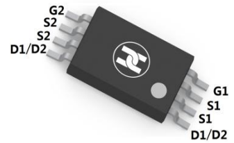
TSSOP-8
