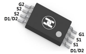
TSSOP-8
