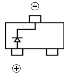
SOT-323
