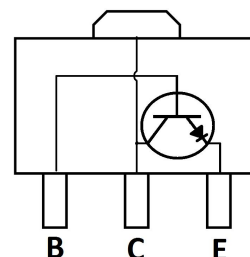
SOT-89
